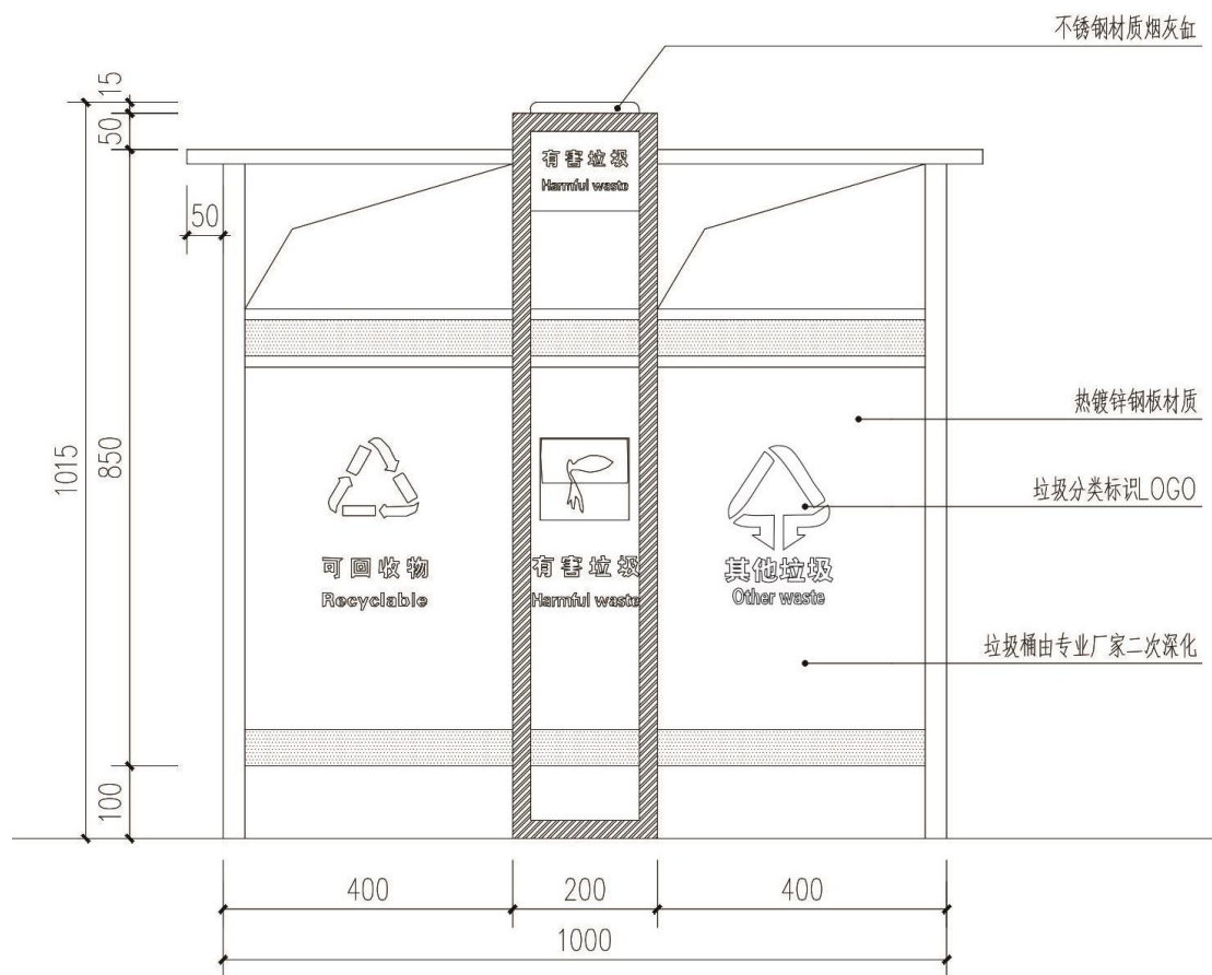
图 2: 废物箱正面参考示意图
