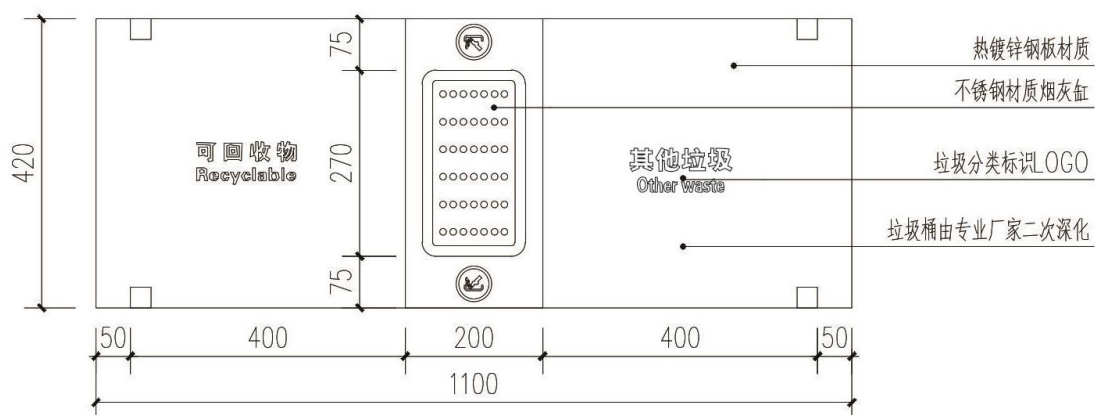
图 1: 废物箱顶部参考示意图
