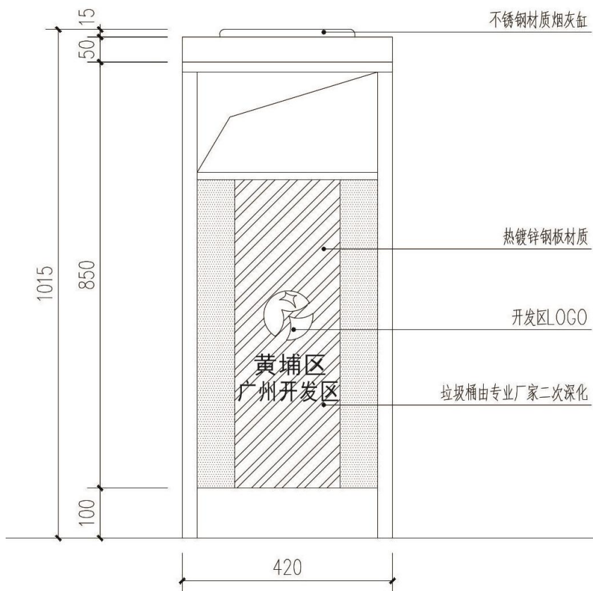
图 3: 废物箱侧面参考示意图
